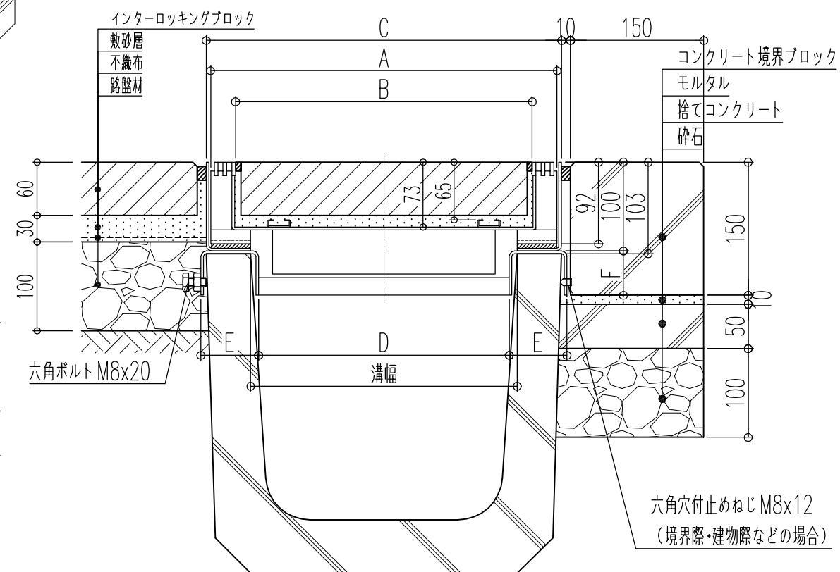
施工参考図
